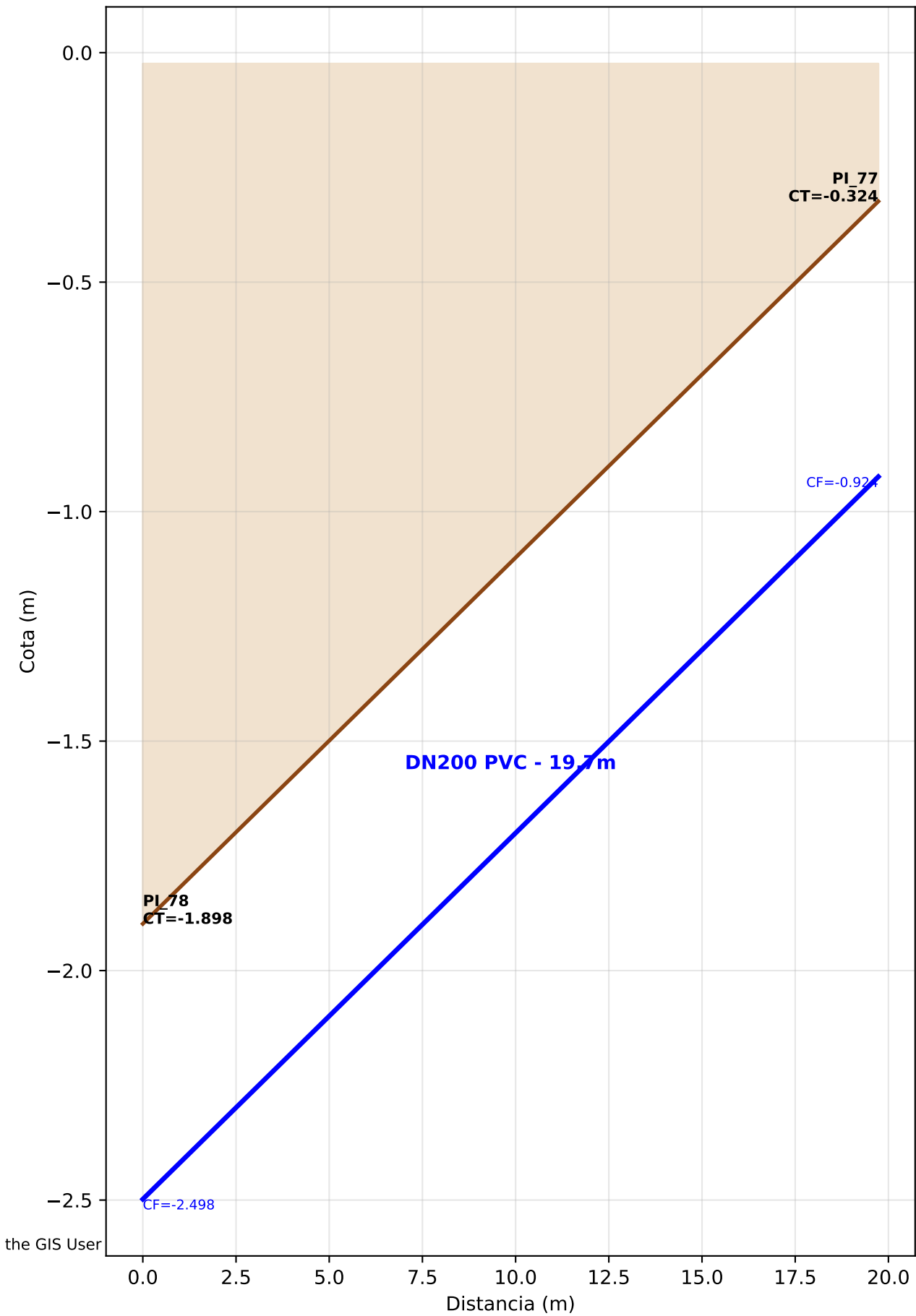
PERFIL LONGITUDINAL - NS 060
